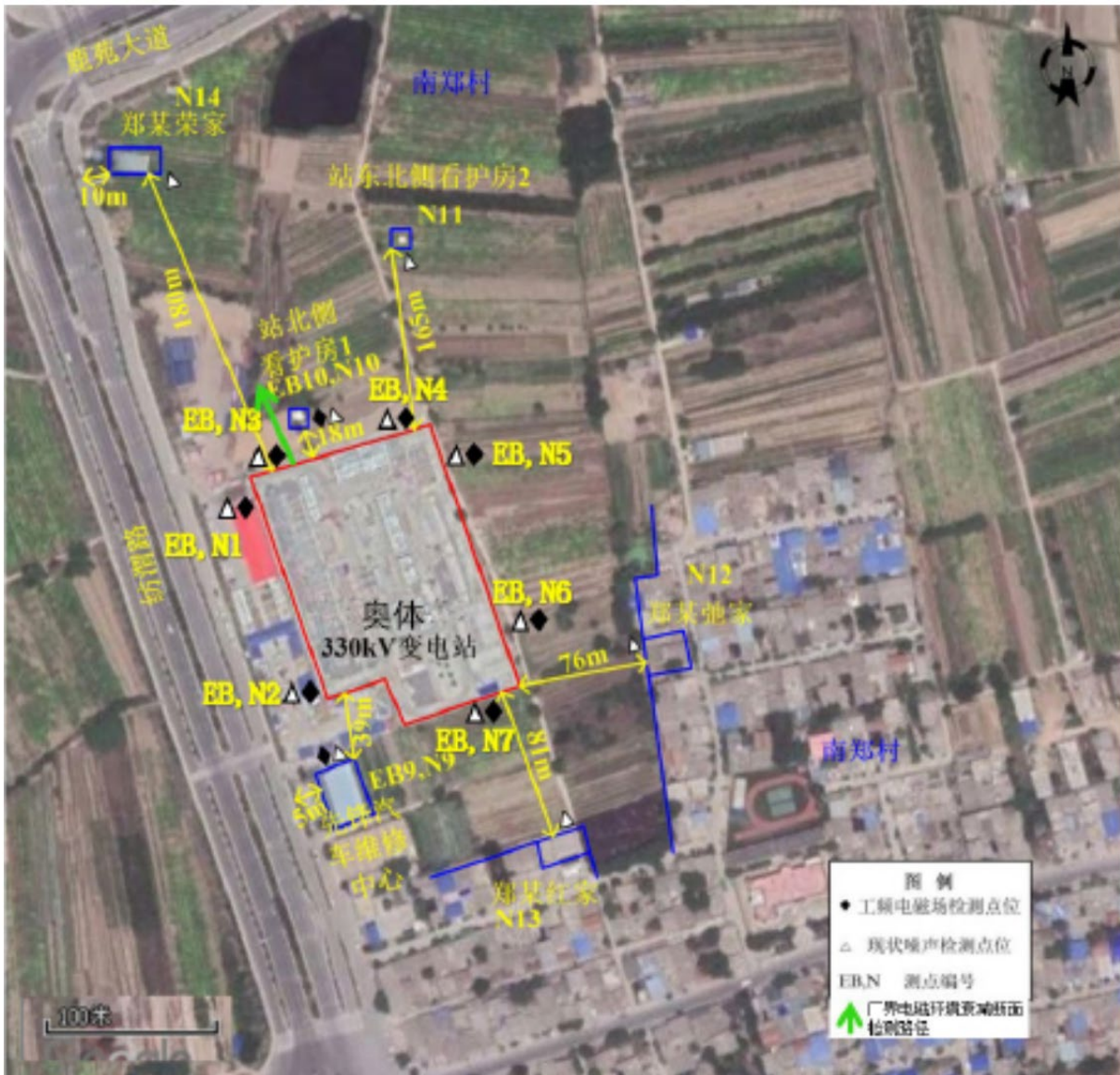
图 10 奥体 330kV 变电站厂界及环境敏感目标监测布点示意图
