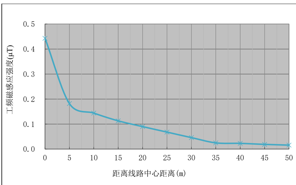
图 12 330kV 奥体变电站断面监测工频磁感应强度分布图
