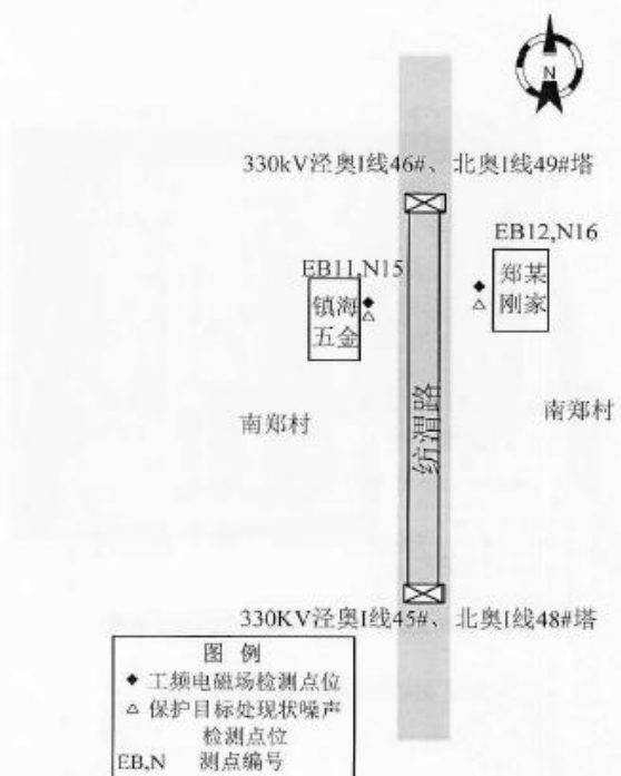
图3 330kV 泾奥 I 线、北奥 I 线调查范围内的保护目标检测点位示意图（南郑村）
