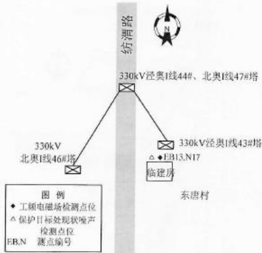
图 4 330kV 泾奥 I 线、北奥 I 线调查范围内的保护目标检测点位示意图（东唐村）
