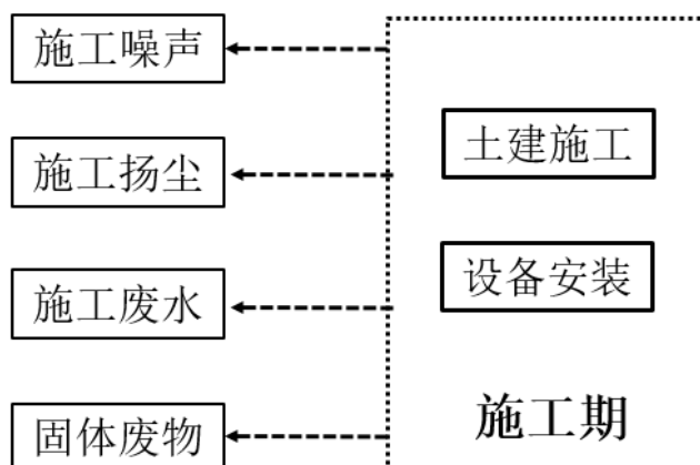
图 6 变电站间隔扩建工程施工期产污节点图
