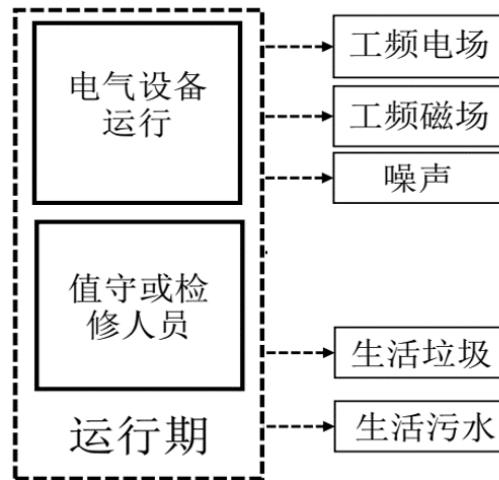
图8 变电站运营期产污节点图
