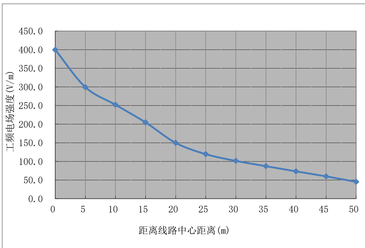
图 11 330kV 奥体变电站断面监测工频电场强度分布图
