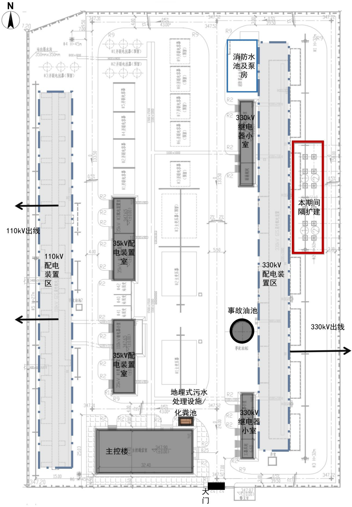
附图 3: 330kV 春光变电站总平面图
